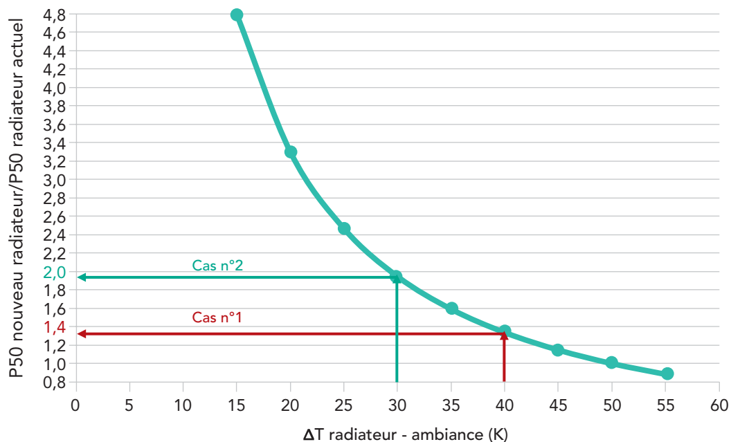
Figure 5 : Détermination de la puissance P50 des nouveaux radiateurs en fonction du \Delta T prévu pour le redimensionnement des radiateurs
