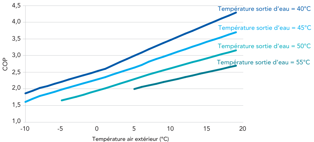
Figure 2 : Evolution du COP en fonction de la température extérieure et pour différents températures de sortie d'eau
