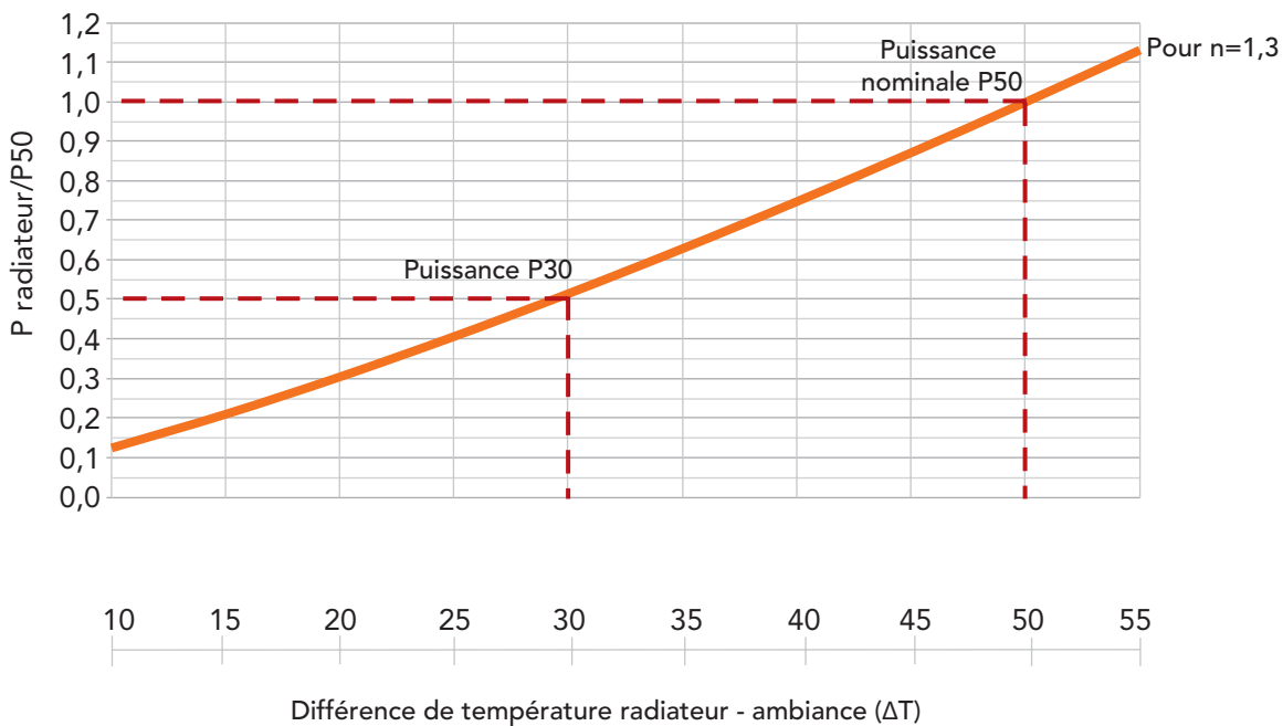
Figure 4 : variation de la puissance P du radiateur (par rapport à P50) en fonction de la différence de température ( \Delta T ) entre la température moyenne de l'eau et la température d'ambiance (avec une pente d'émission (n) de 1,3).
