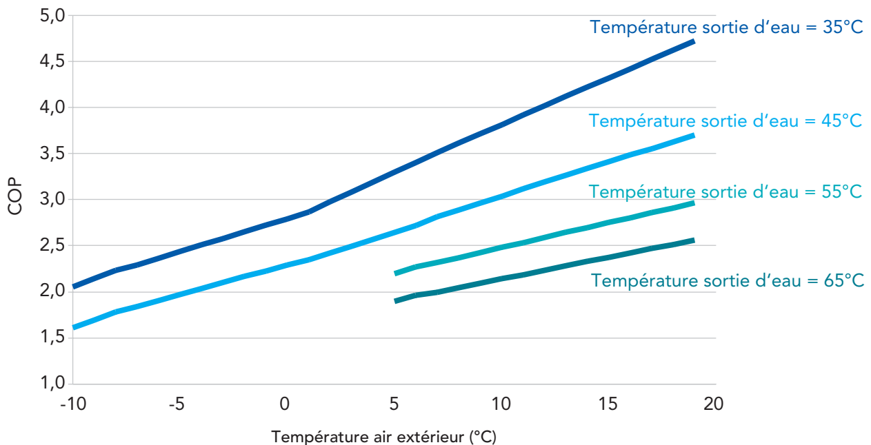
Figure 3 : Exemple pour une PAC air/eau de plages d'utilisation en fonction de la température de sortie d'eau et de la température extérieure
