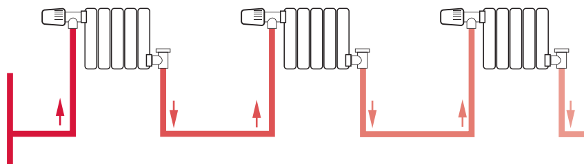
Schéma simplifié d'une installation monotube série
